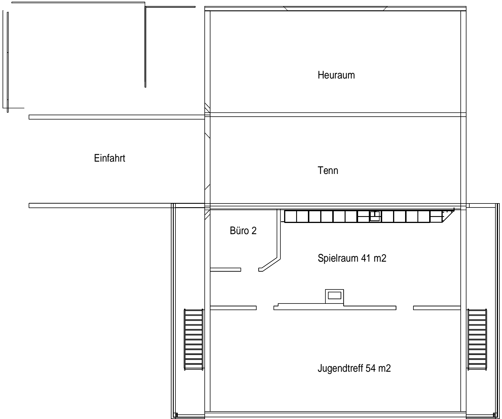
1.Obergeschoss
